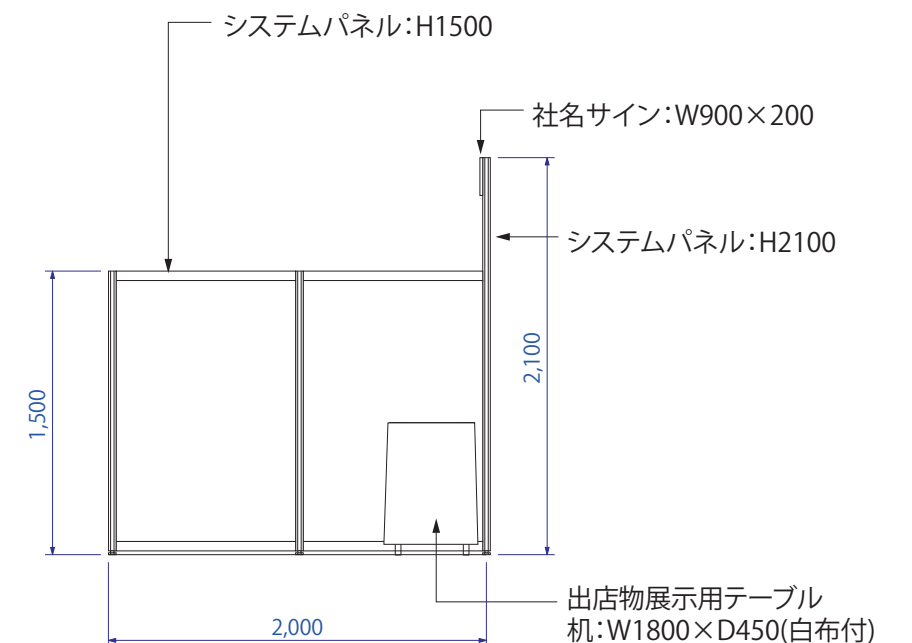
側面図
