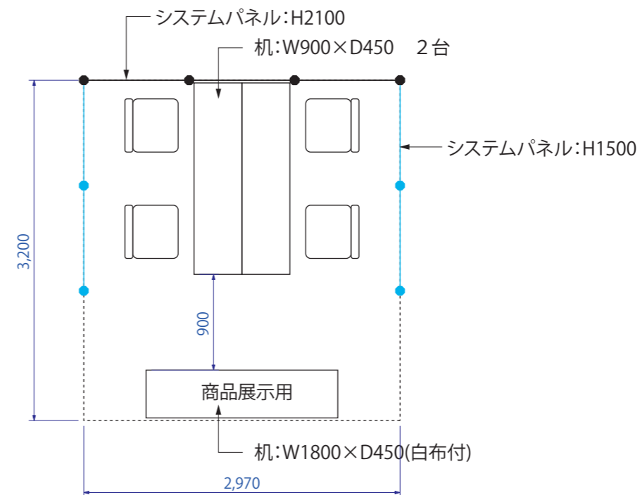
A-2:バックシステムパネルH2100タイプ 平面図
